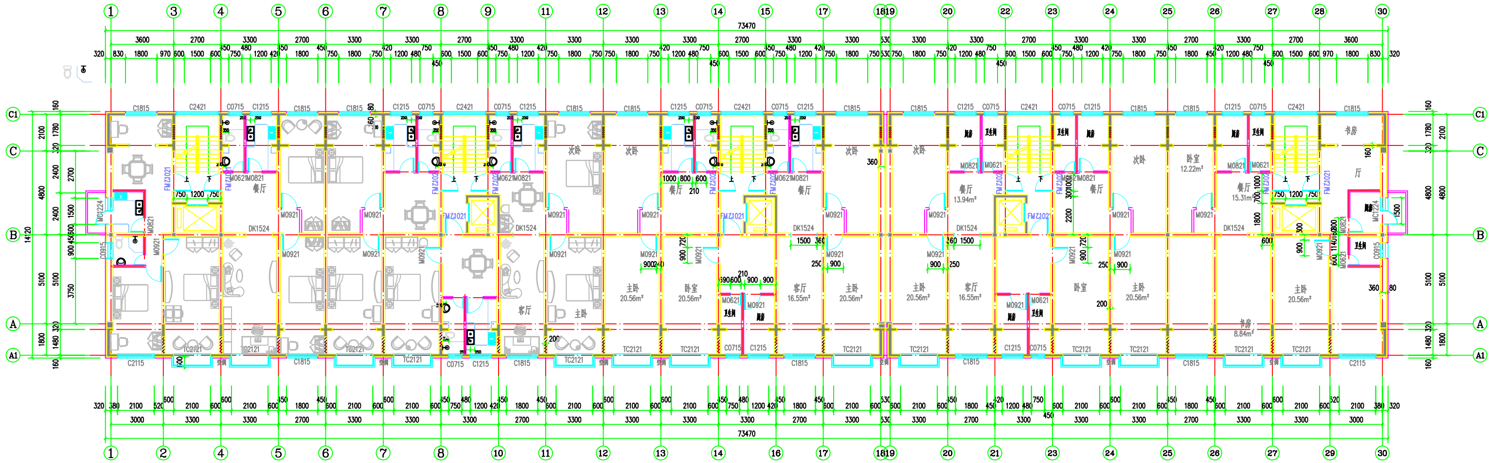
标准层平面图 1:100
